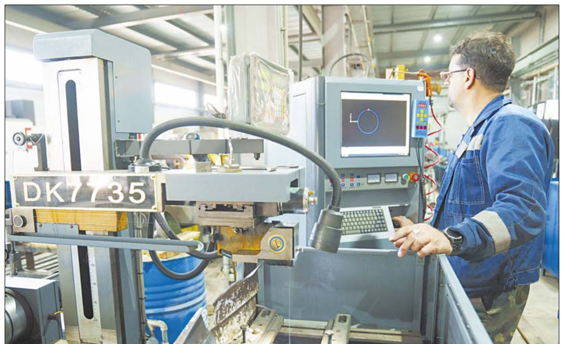
При помощи электрических разрядов, проходящих через проволоку, можно обрабатывать заготовки из материалов высокой твердости.
