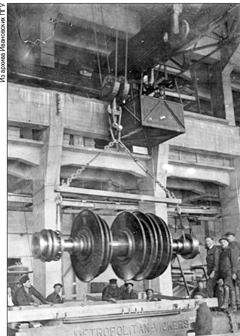
Установка ротора турбины.
